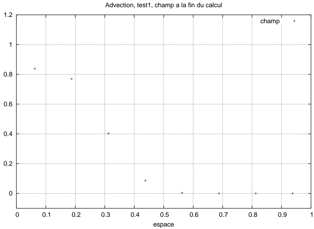
Figure 1 advection, 8 mailles, pas d'extrapolation
